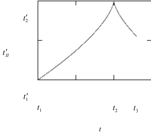
Fig. 3. Representación gráfica de t'_{II} frente a t para r fijo durante la segunda etapa del viaje temporal
