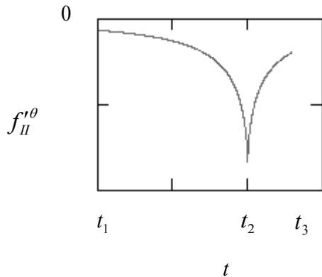
Fig. 6. Representación gráfica de f_{II}^{r'\theta} frente a t para r fijo durante la segunda etapa del viaje temporal.
