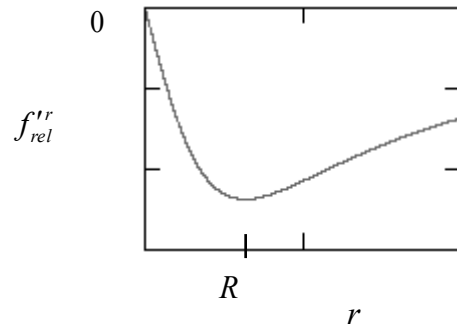
Fig. 2. Representación gráfica de f'_{rel}{}^r frente a r a velocidad angular \omega constante.
