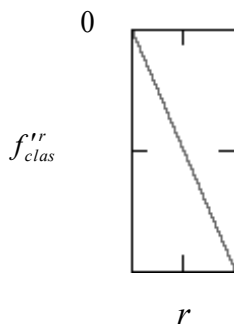
Fig. 1. Representación gráfica de f'_{clas} frente a r a velocidad angular \omega constante.
