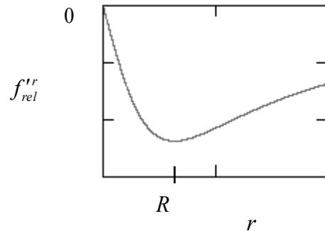
Fig. 2. Representación gráfica de f'_{rel} frente a r a velocidad angular \omega constante.
