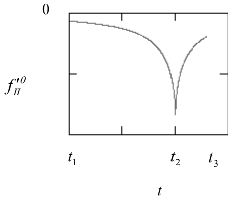
Fig. 6. Representación gráfica de f_{II}^{\prime\theta} frente a t para r fijo durante la segunda etapa del viaje temporal.
